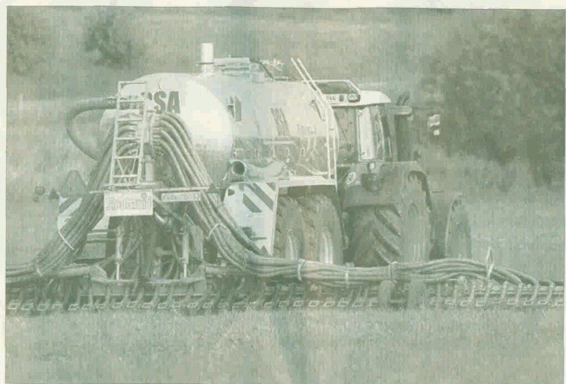
So sieht moderne Landwirtschaft aus: Vorführung eines Schlitzkufenverteilers, der zwischen Kottspiel und Bühlerzell Gülle ausbringt. Foto: Weigert
